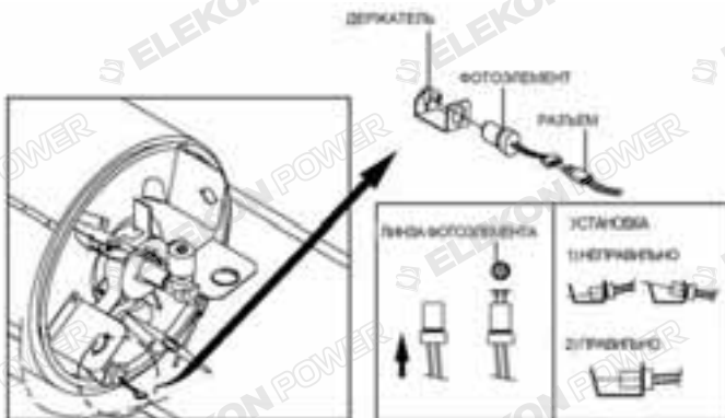
Рис. 11. Фотоэлемент
