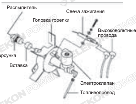
рис. 10 Форсунка
