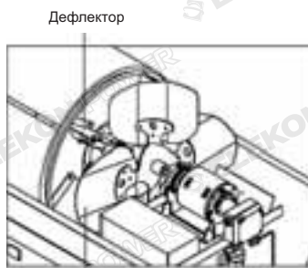
Рис 8. Лопасть вентилятора и дефлекторы
