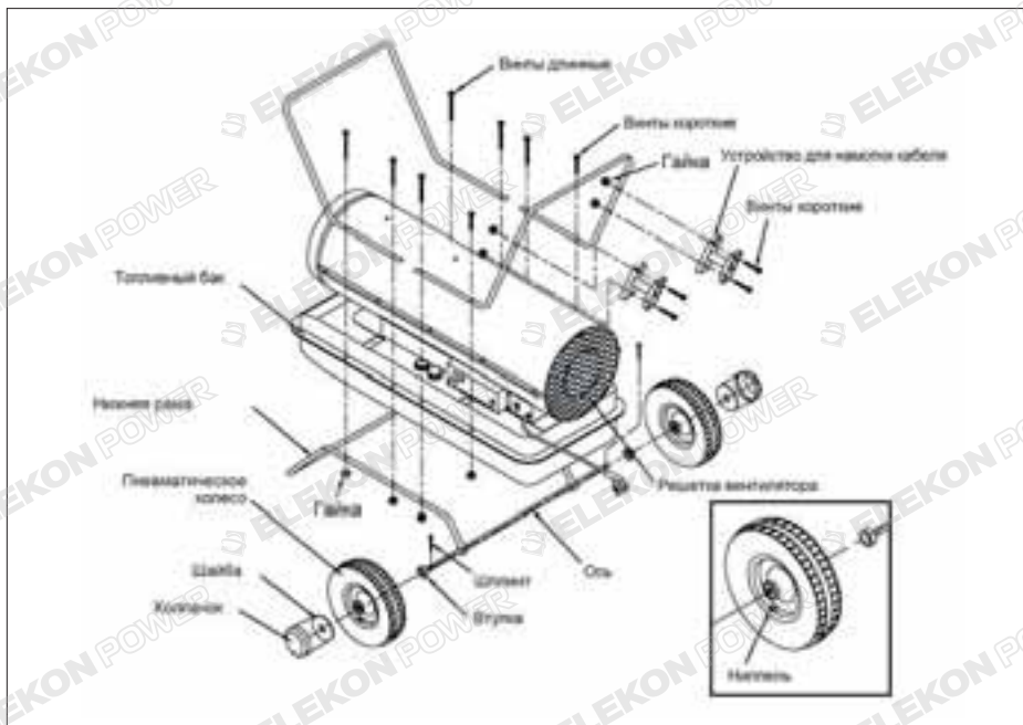
Рис 3. Сборка нагревателя
